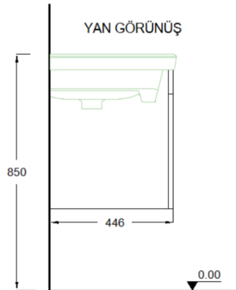
VENTO 100 CM LAVABO DOLABI
