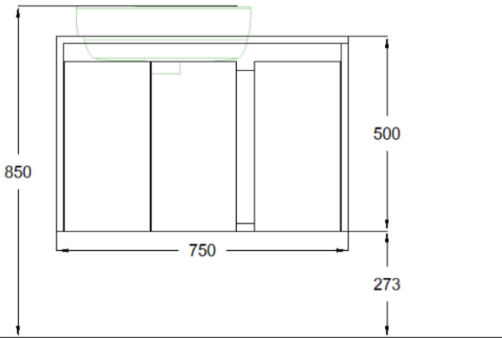
ÖN GÖRÜNÜŞ
